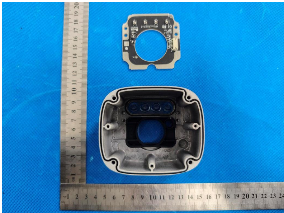
EUT PHOTO 15
