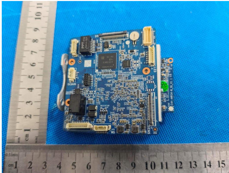
EUT PHOTO 25
