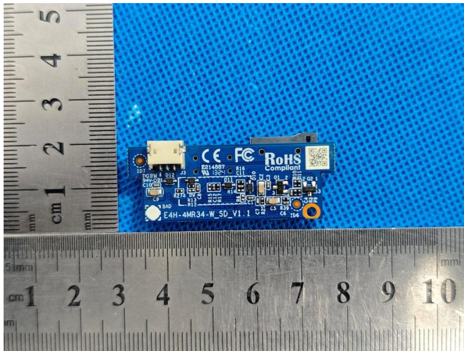
EUT PHOTO 29
