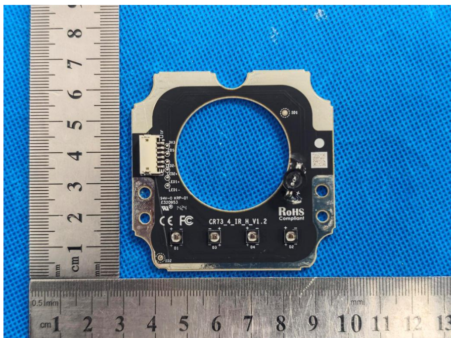
EUT PHOTO 16
