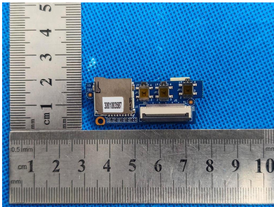
EUT PHOTO 30
