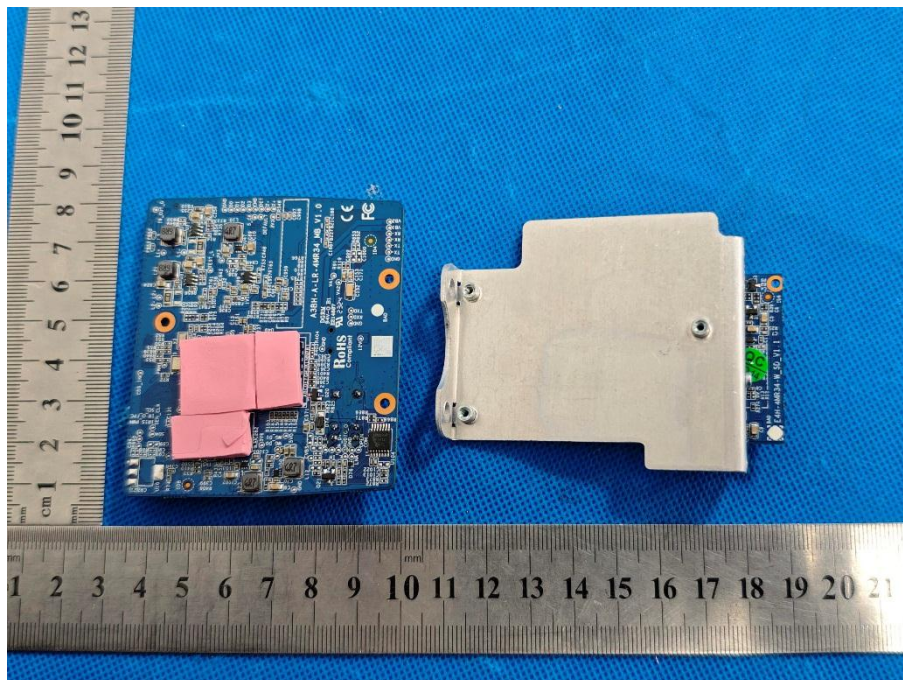
EUT PHOTO 26
