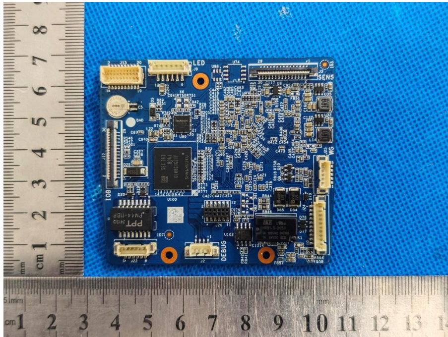
EUT PHOTO 27
